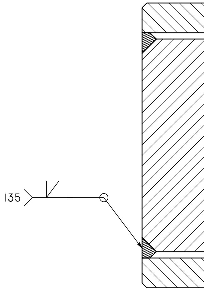
A-A ( 2 : 1 )
