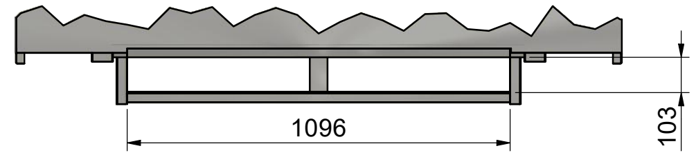
A-A ( 1 : 15 )
